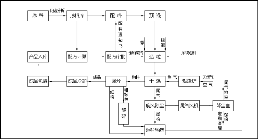
图 5-5 自产复合肥生产工艺流程图
